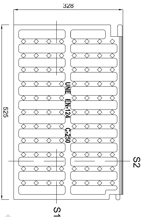
TAPA. VISTA SUPERIOR.
